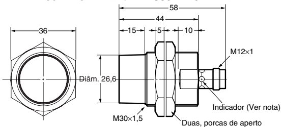
E2A-M30KN20-M1-□□/E2A-S30KN20-M1-□
