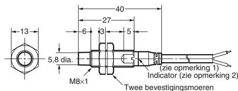
E2A-S08KN04-WP-□□
