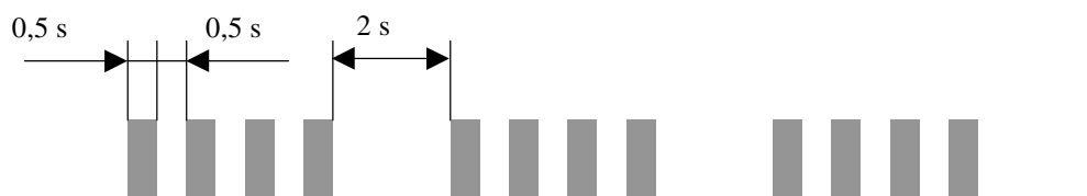
Fig. Diagramma della frequenza dei lampeggi della spia rossa
