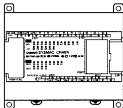
UC à 20/30 points entrée/sortie
