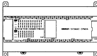
UC à 60 points d'entrée/sortie
