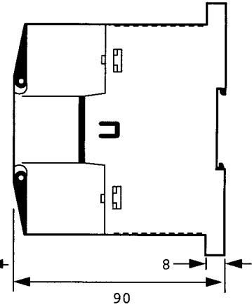
UC avec alimentation alternative
